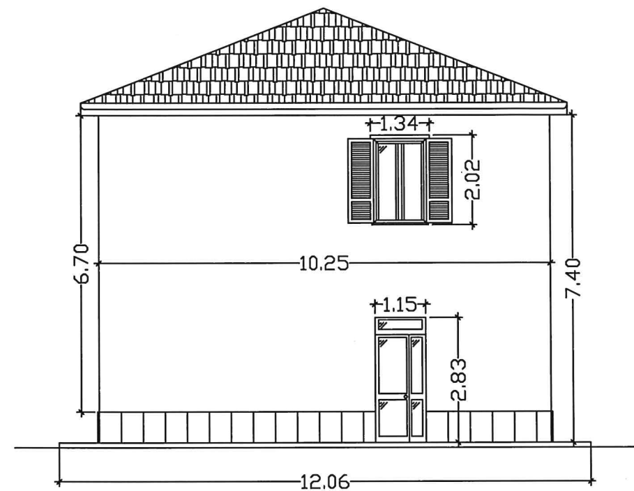
PROSPETTO LATO OVEST facciata mq 63.22
