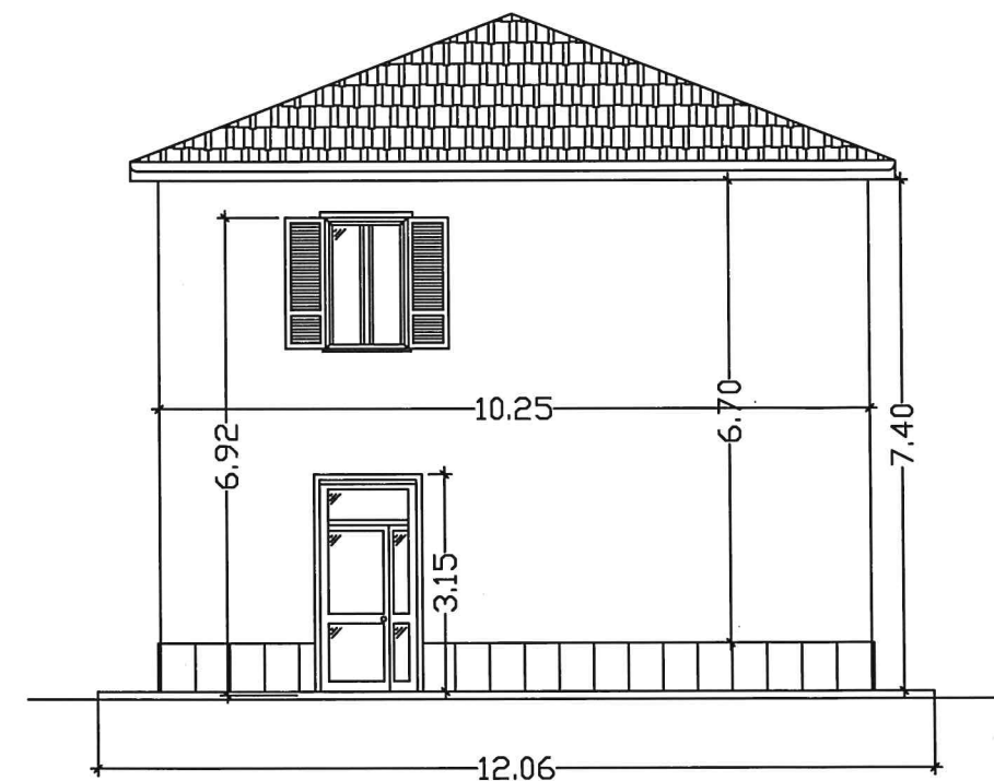
PROSPETTO LATO EST facciata mq 63.22
