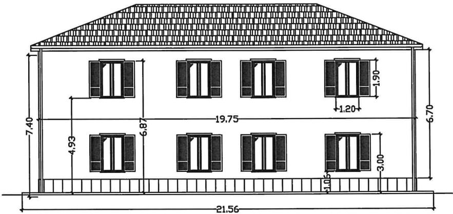
PROSPETTO LATO NORD facciata mq 114.08
