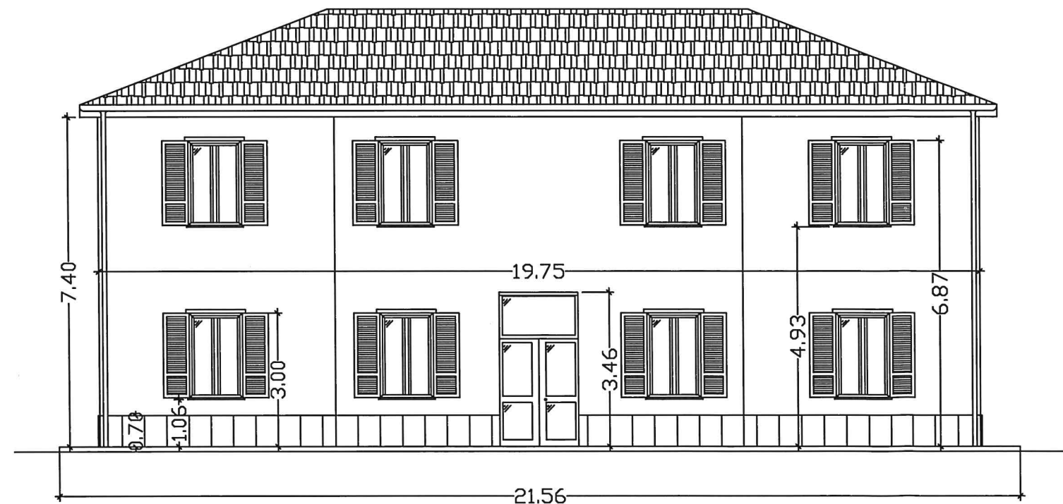
PROSPETTO LATO SUD facciata mq 125.28
