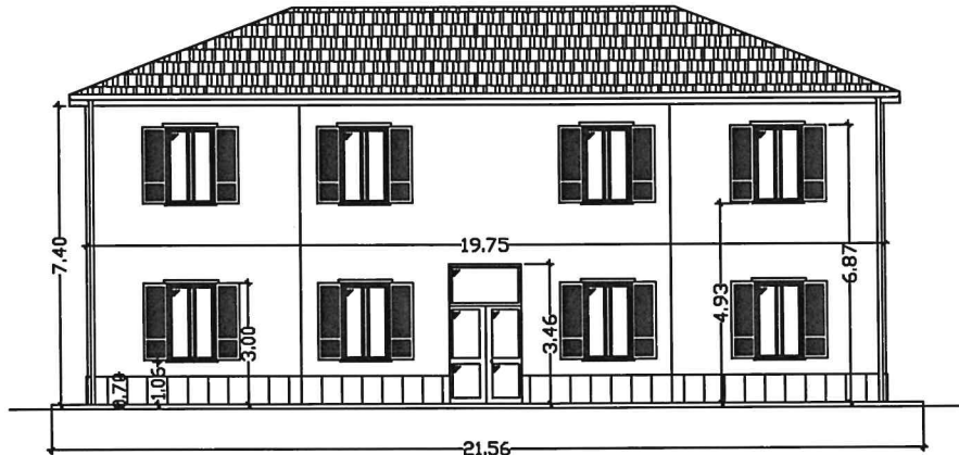
PROSPETTO LATO SUD facciata mq 125.28
