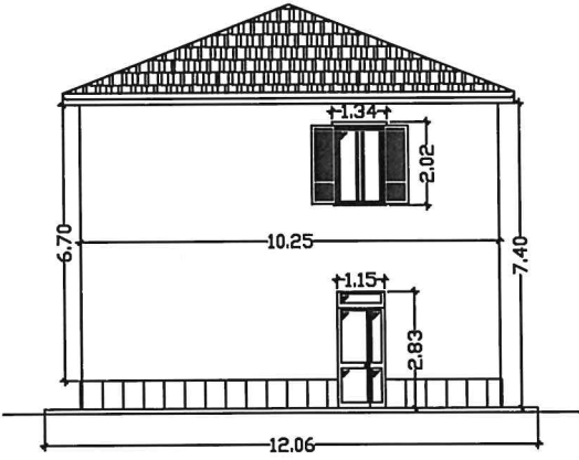
PROSPETTO LATO OVEST facciata mq 63.22
