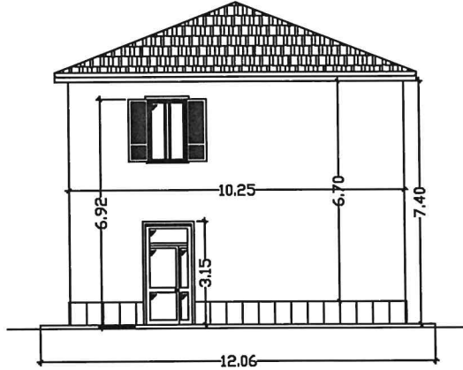
PROSPETTO LATO EST facciata mq 63.22
