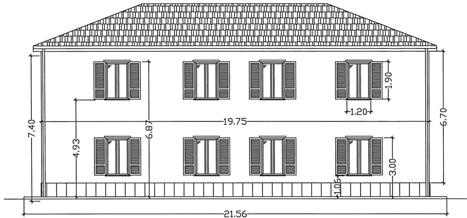
PROSPETTO LATO NORD facciata mq 114.08
